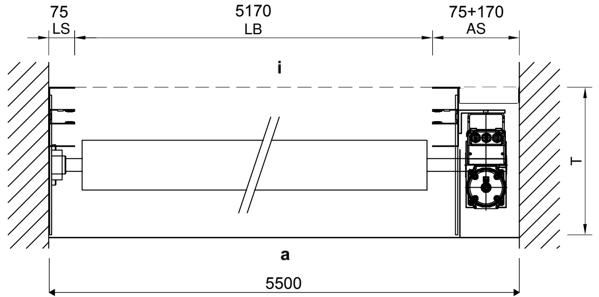
Detail Führungsschiene/ detail side guide
