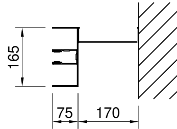
Detail Führungsschiene/ detail side guide
